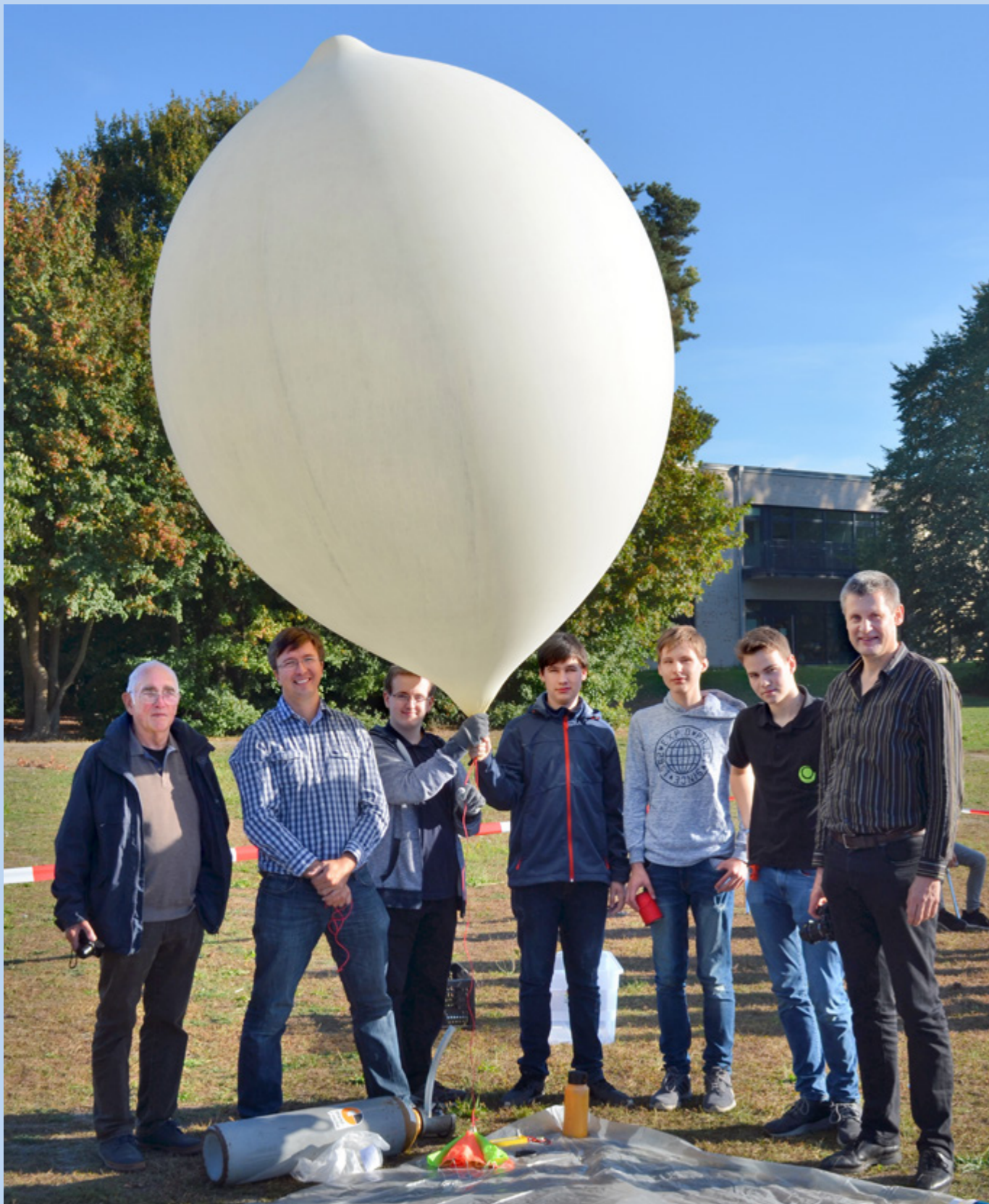
Gemeinsames Experimentieren beim Wetterballontest
